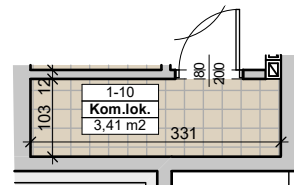
Komórka lokatorska 1-10
