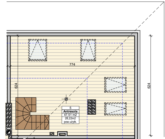
POZIOM GÓRNY (ANTRESOLA)
