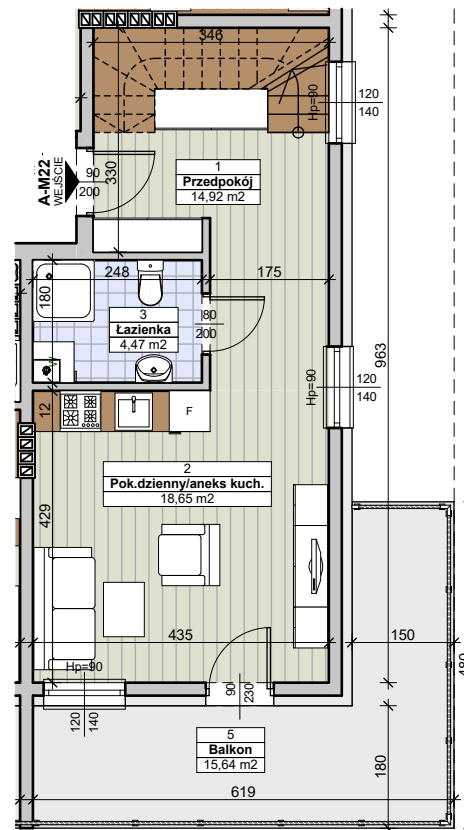
POZIOM DOLNY
