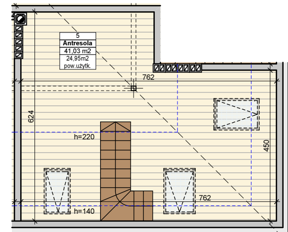
POZIOM GÓRNY (ANTRESOLA)
